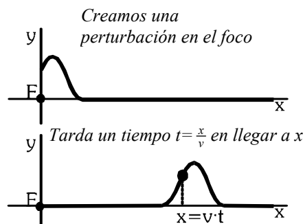
La perturbación en el pto x será la que tenía el foco hace algunos segundos ( t = \frac{x}{v} )
