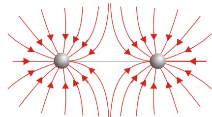
Líneas de campo gravitatorio generado por dos masas puntuales iguales.
