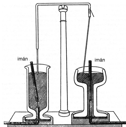
Figura 26 - Rotor electromagnético de Faraday [8].
