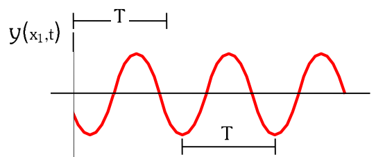
Elongación de un punto x_1 del medio en función del tiempo.
