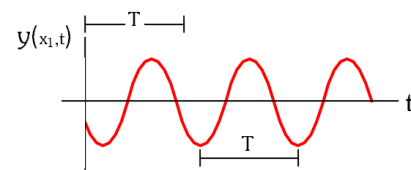
Elongación de un punto x_1 del medio en función del tiempo.
